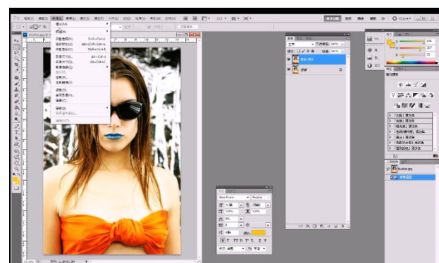
2 複製圖層
