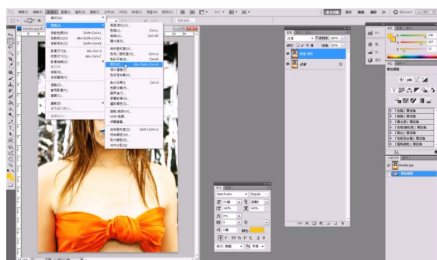
3.到影像→調整
