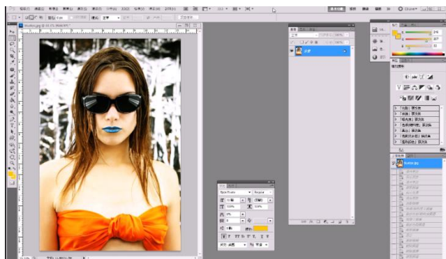
1 打開圖檔
